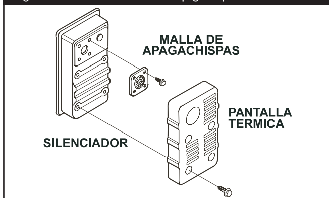
Figura 25 — Servicio al Pantalla Apagachispas
